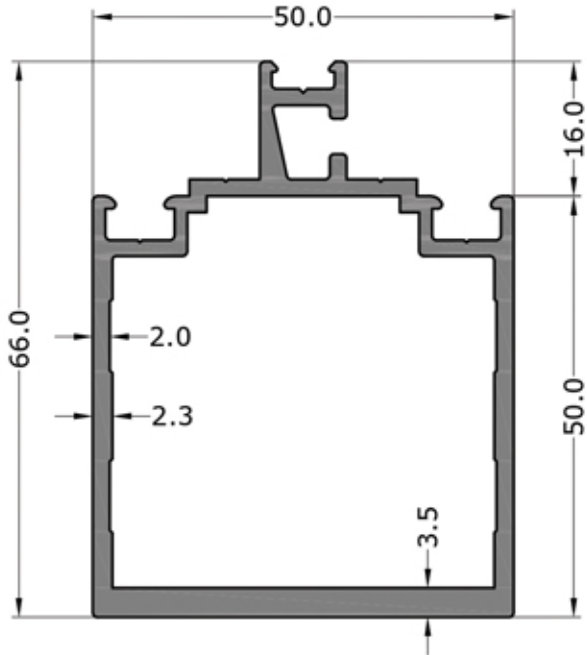
3168 1.478 KG/M
