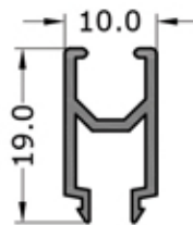
1181 0.159 KG/M
