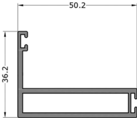
3264 0.759 KG/M (2.0 MM)
