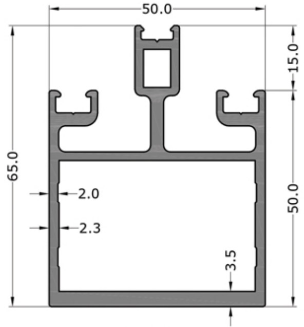
3169 1.795 KG/M
