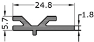
1130 0.201 KG/M
