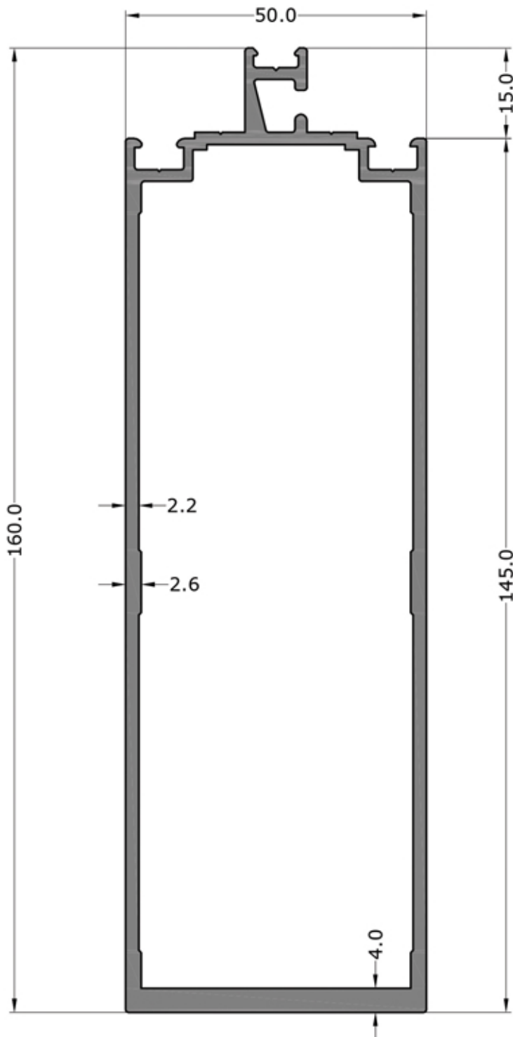
3317 2.714 KG/M
