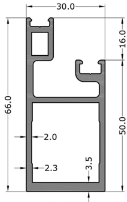
3254 1.305 KG/M
