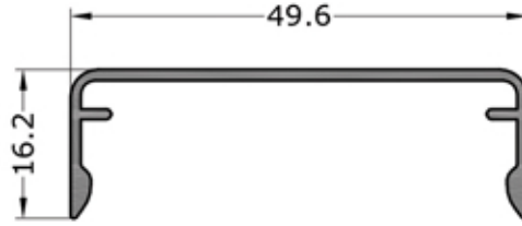
1182 0.280 KG/M
