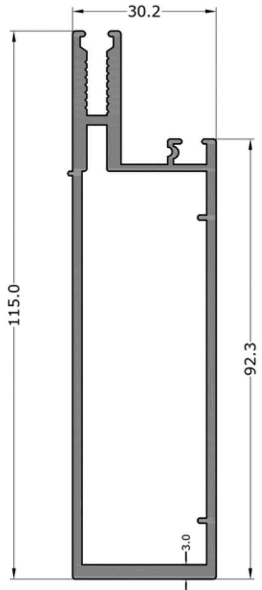
3267 1.748 KG/M (2.0 MM)
