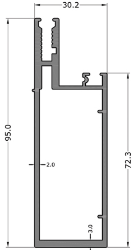
3263 1.522 KG/M (2.0 MM)
