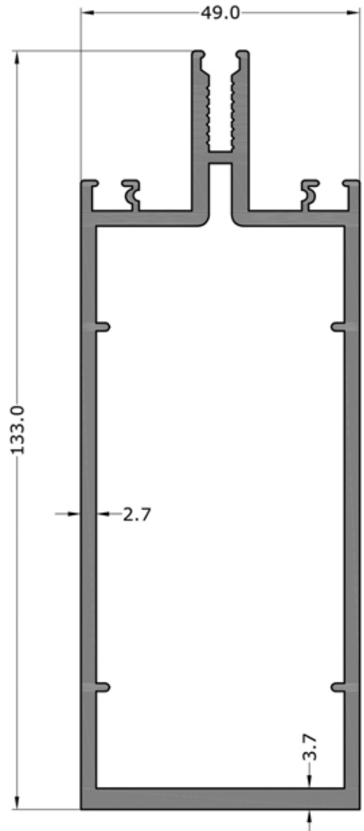
3277 2.834 KG/M (2.7 MM)
