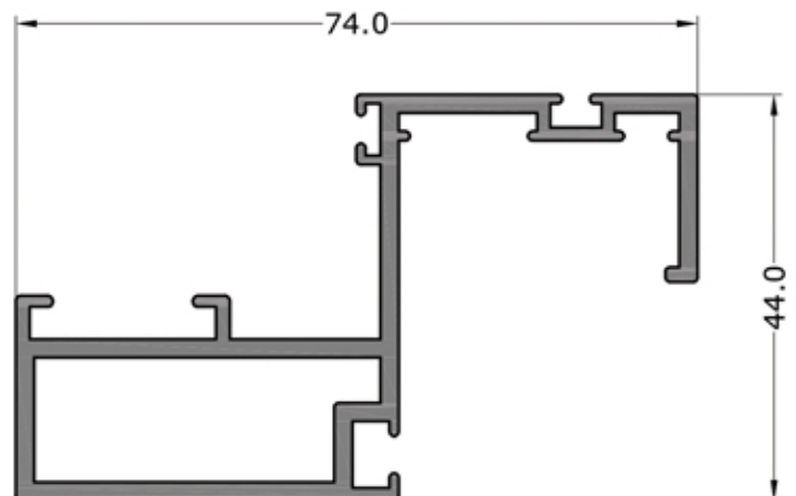
3332 1.147 KG/M (2.0 MM)
