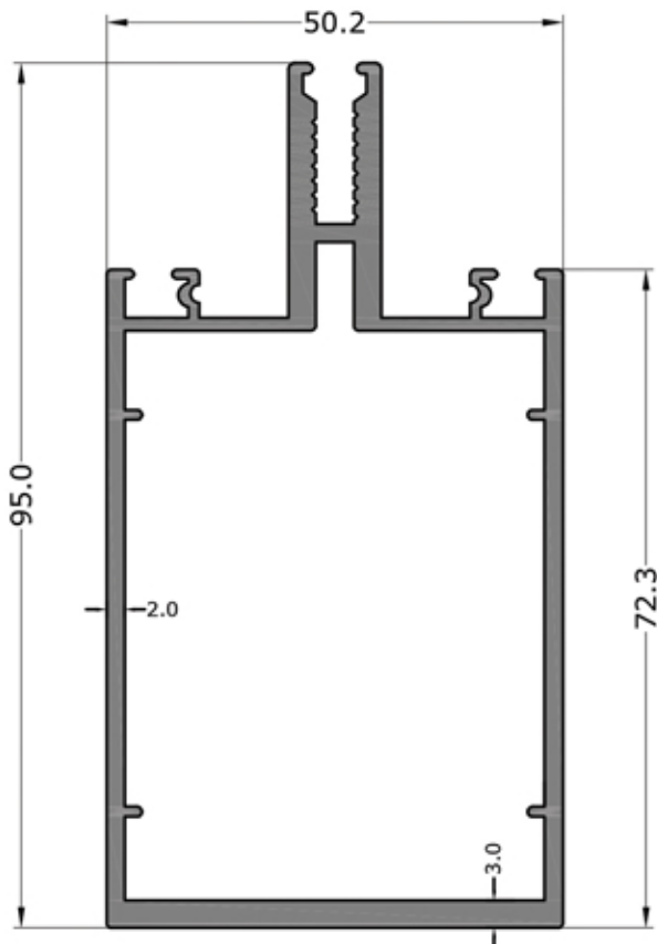
3262 1.832 KG/M (2.0 MM)
