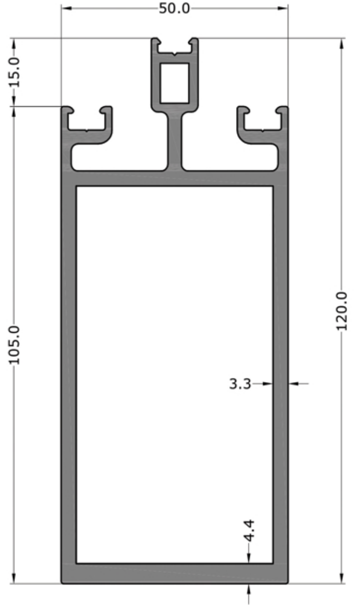
3291 3.211 KG/M
