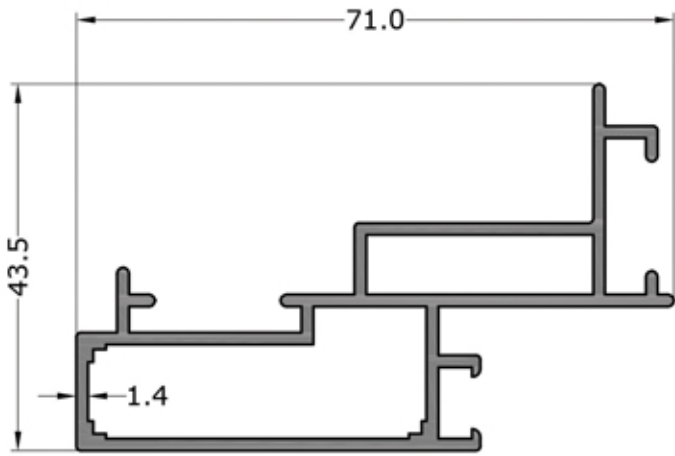
3186 0.928 KG/M
