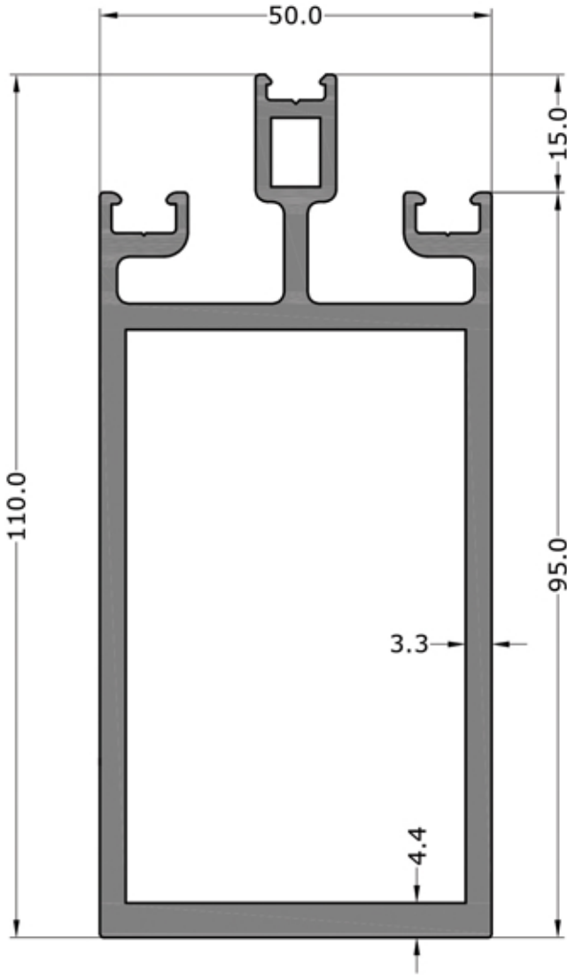
3290 3.033 KG/M
