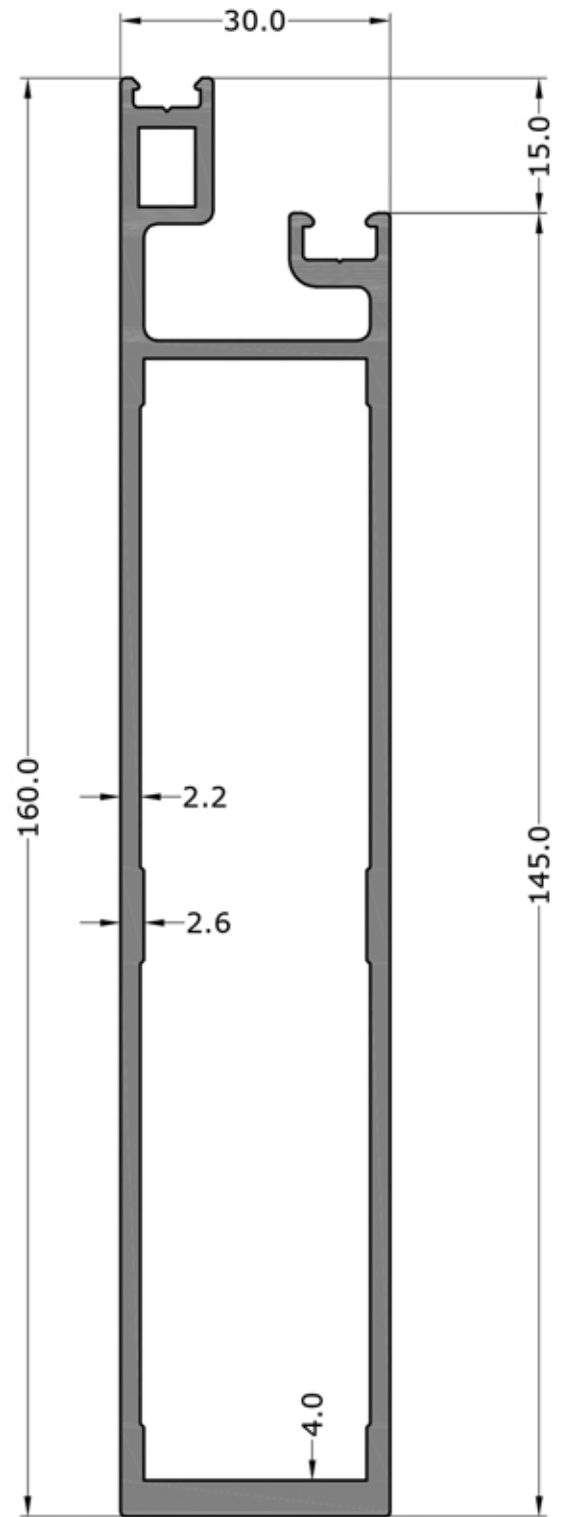
3316 2.517 KG/M
