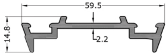
1056 0.557 KG/M
