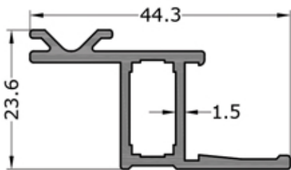
3187 0.478 KG/M
