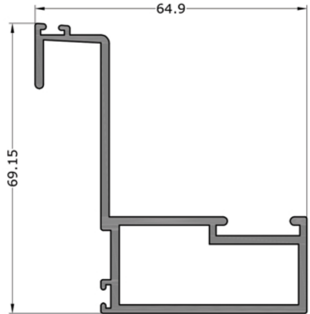
3265 1.175 KG/M (2.0 MM)
