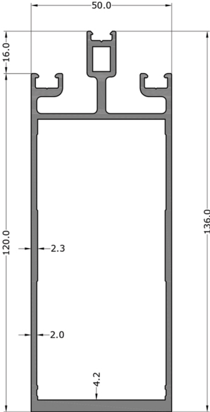
3325 2.650 KG/M
