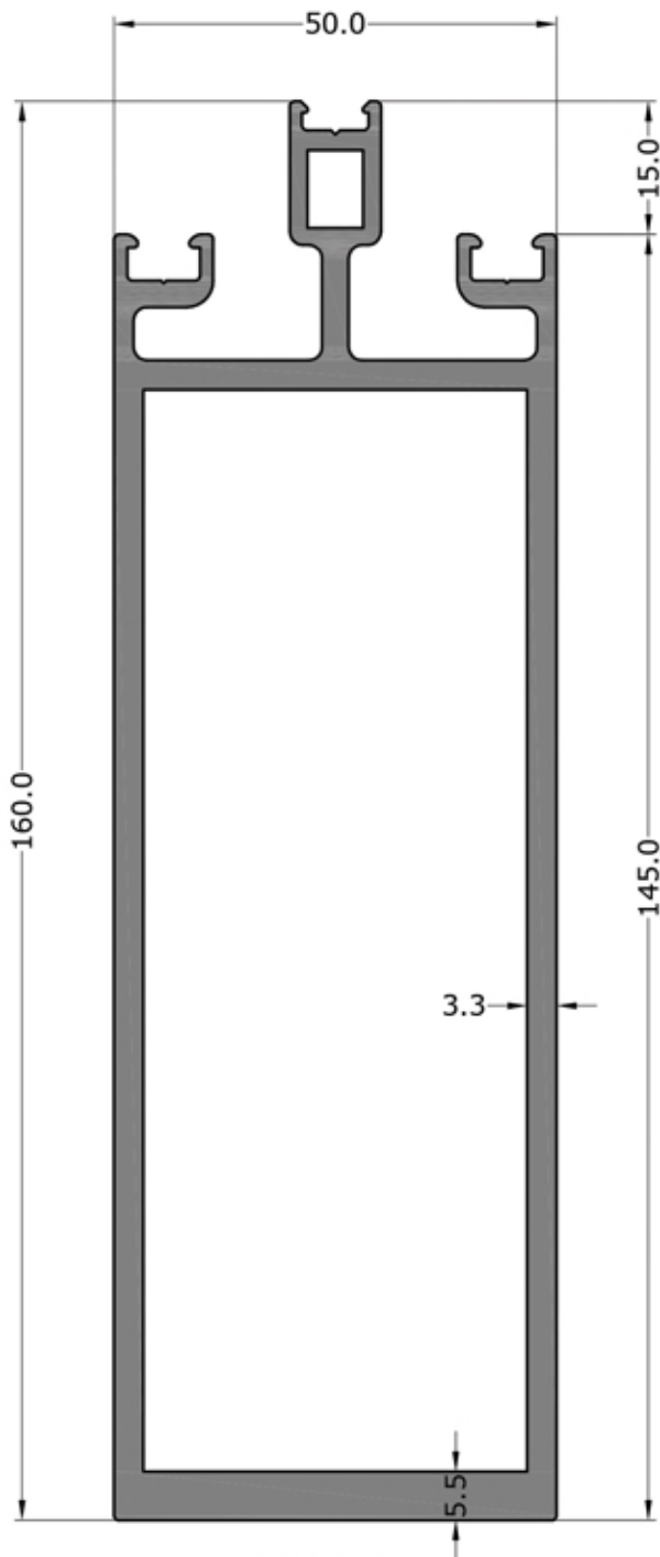
3292 4.052 KG/M
