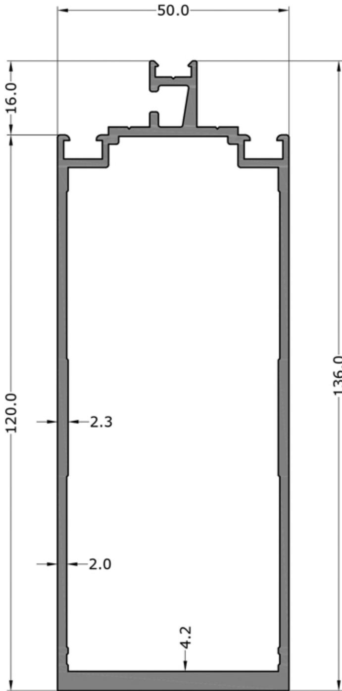
3323 2.315 KG/M
