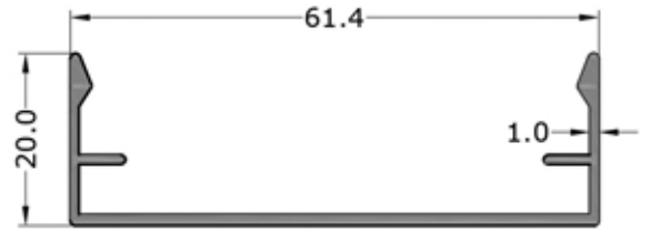
1054 0.362 KG/M
