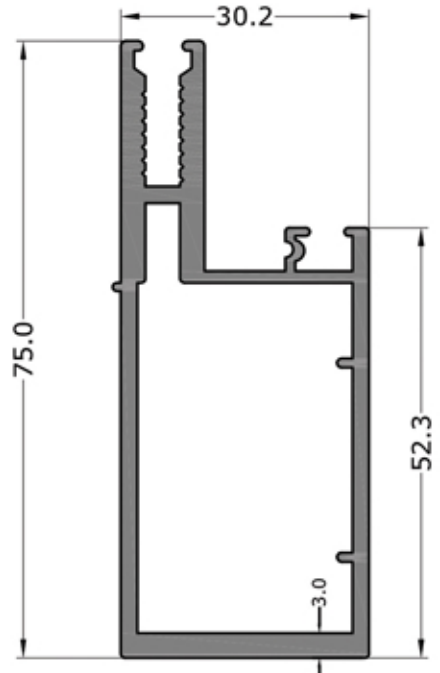
3269 1.316 KG/M (2.0 MM)
