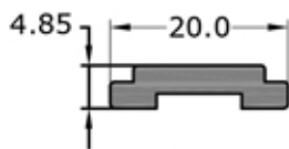
1099 0.182 KG/M
