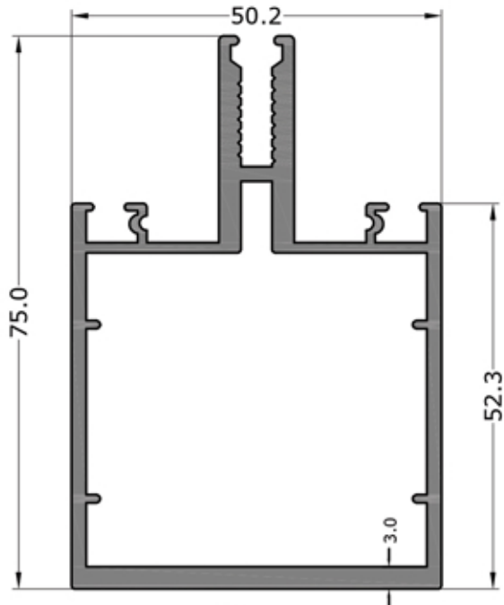
3268 1.616 KG/M (2.0 MM)
